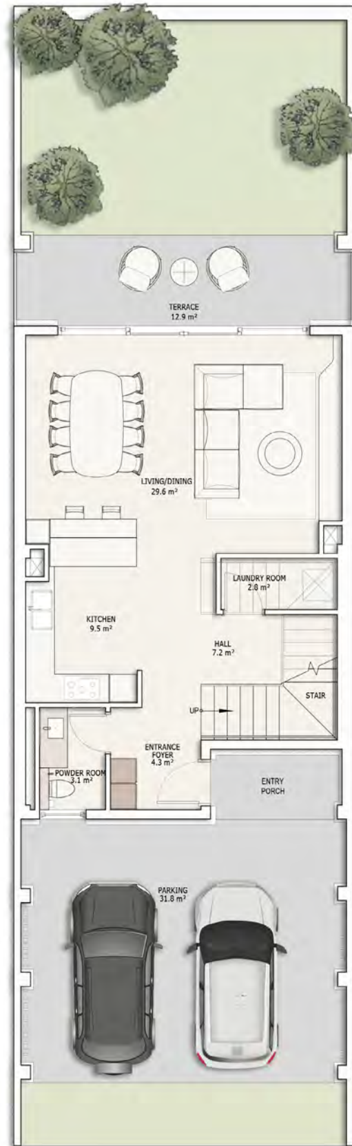
План первого этажа
